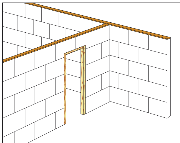
Désolidarisation en tête par bande résiliente.
